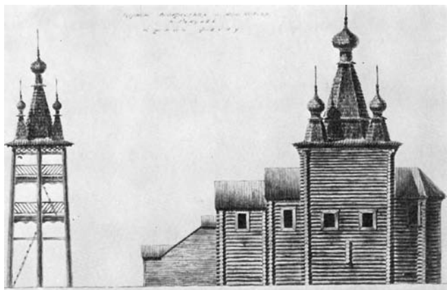
Ракула. Колокольня и Воскресенская церковь. Реконструкция первоначального облика по обмерам П. Барановского, И. Рильского, Ю. Гребенщикова, 1936
